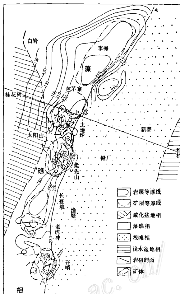
图1 鱼塘寨铅锌矿与岩相关系图
