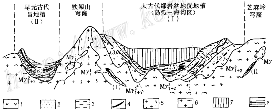
图2 鞍山本太古代绿岩盆地成矿模式图
