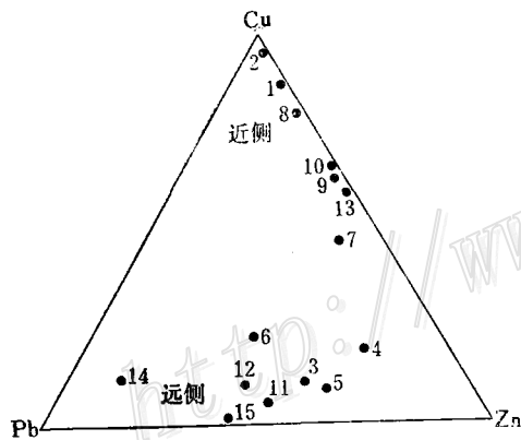
图3 祁连地槽主要块状硫化物矿床金属组分比例关系图
