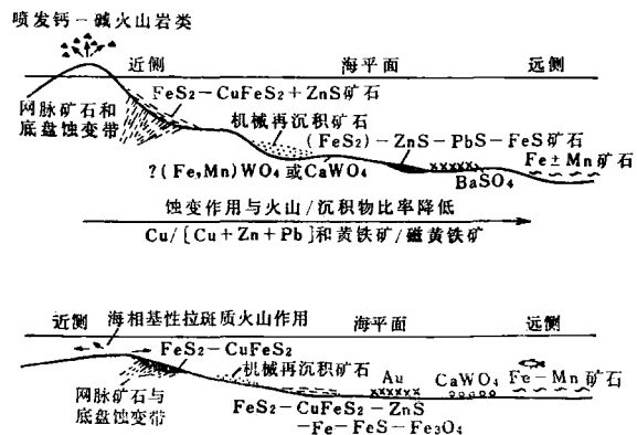
图4 与拉斑质和钙碱质火山岩系列有关的近侧与远侧矿床形成空间关系图 (据Plimer, 1978)
