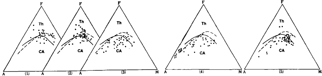
图 1 北祁连优地槽带各区段火山岩A-F-M组分变化图
