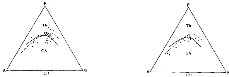
图2 南祁连优地槽带各区段火山岩A-F-M组分变化图
