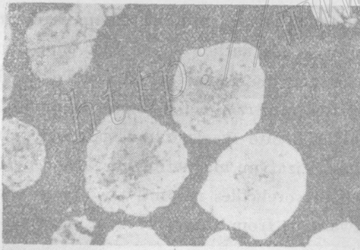
5、铅锌矿石交代和胶结锰铝榴石呈似海绵陨铁结 构，黑色为铅锌矿 单偏光 32 东风矿段
