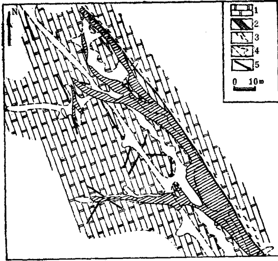
图3 东风矿段155m中段交代脉状矿体示意图 (据辽宁冶金五队)
