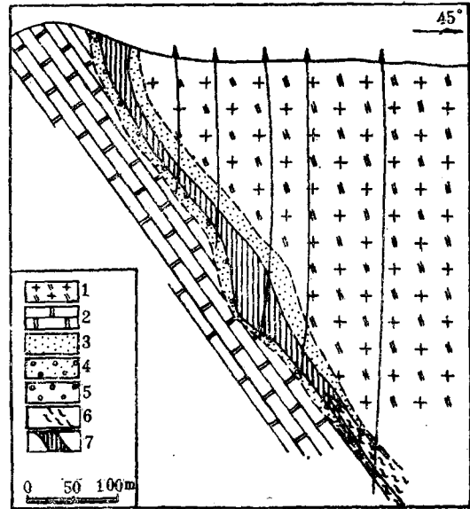
图4 北山矿段49线剖面矿化蚀变分带示意图 (据辽宁三队)
