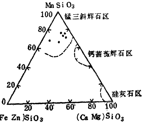
图8 MnSiO 3 -FeSiO 3 -CaSiO 3 成分关系图 Fig. 8. Triangular diagram of MnSiO 3 -FeSiO 3 -CaSiO 3 .
