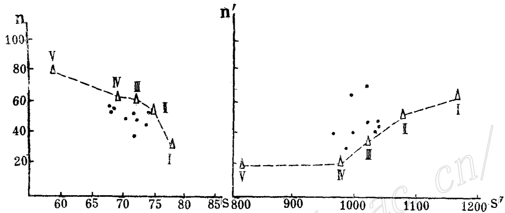
图2 黑云石英闪长岩n—S、n'—S'图解 (仿胡受奚, 1982)
