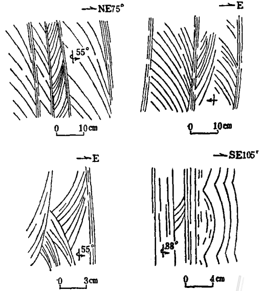
图2 裴家庄组中的原生沉积构造 (示斜交层理和波痕)
