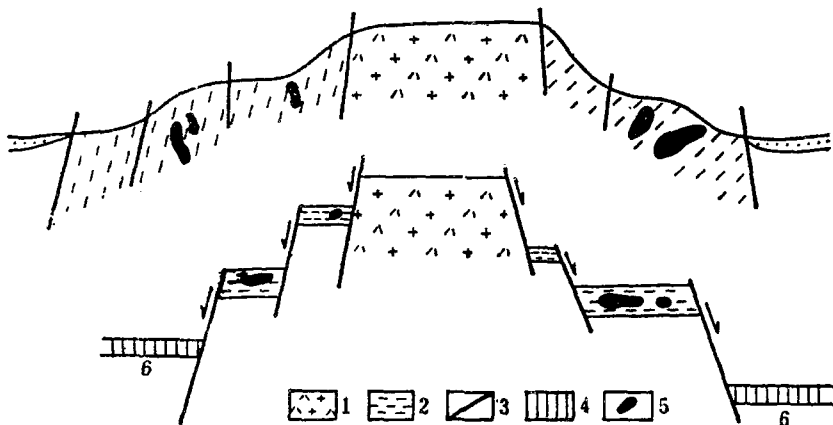
图6 霍格气—炭窑口剖面多金属矿床与断陷带关系
