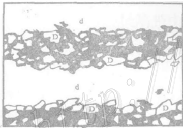
图1 铜矿物与粗粒、重结晶白云石共生关系素描图（单偏光 ×25）
