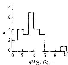
图4 支家地银矿床硫同位素组成图
