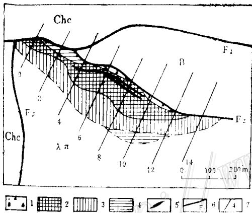
图 2 支家地银矿区隐爆角砾岩筒平面图 \lambda\pi —石英斑岩；B—火山集块岩及火山角砾岩； Chc—含燧石条带白云岩；1—复成分角砾岩； 2—石英斑岩质角砾岩；3—碎裂石英斑岩；4— 崩塌-震碎角砾岩；5—银矿体；6—断层；7— 勘探线
