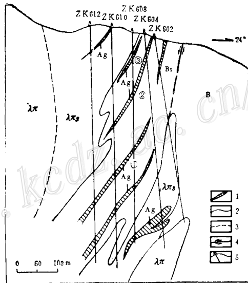
图 3 太白维山支家地银矿区第六勘探线剖面图 \lambda\pi_s —碎裂石英斑岩；Bs—石英斑岩质角砾岩； \lambda\pi —石英斑岩；1—银矿体；2—地质界线；3—推测地质界线； 4—断层；5—钻孔
