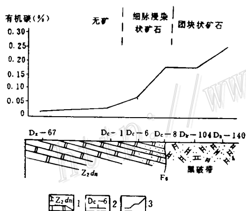
图 4 大梁子矿区地层剖面有机碳含量与铅锌矿化的关系 1—灯影组白云岩; 2—采样位置; 3—有机碳含量变化曲线
