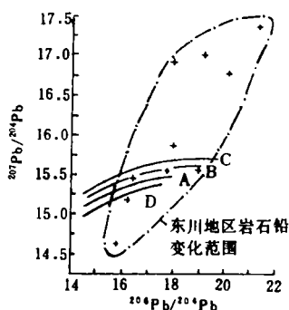
图 7 东川地区昆阳群岩石铅同位素组成特征 (据覃嘉铭等资料改编)
