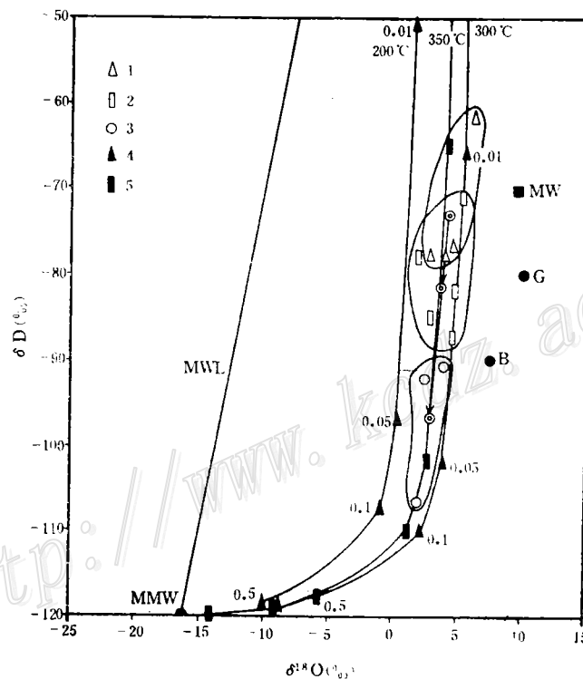
图3 胶东焦家式金矿床不同阶段流体的 \delta D - \delta^{18}\text{O} 变化图
