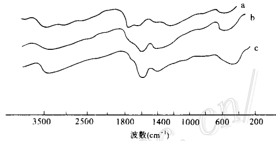
图 2 富啡酸及其铅、锌络合物的红外光谱
