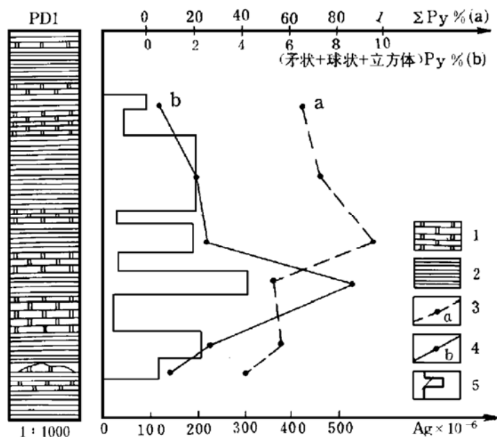
图1 黄铁矿含量与银含量变化曲线图
