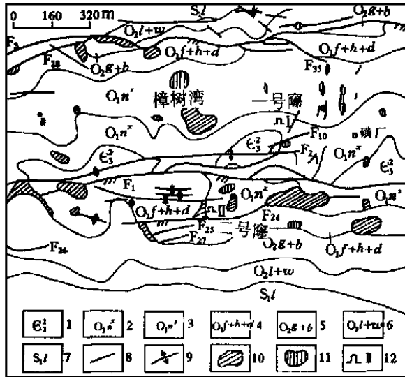
图1 石门雄黄矿一号窿矿区地质图
