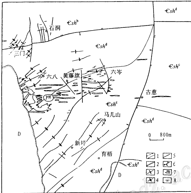
图1 平南北部金矿田地质略图
