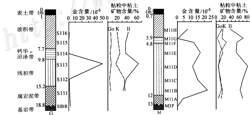
图 3 上芒岗金矿床红色粘土剖面及金和粘粒部分粘土矿物含量
