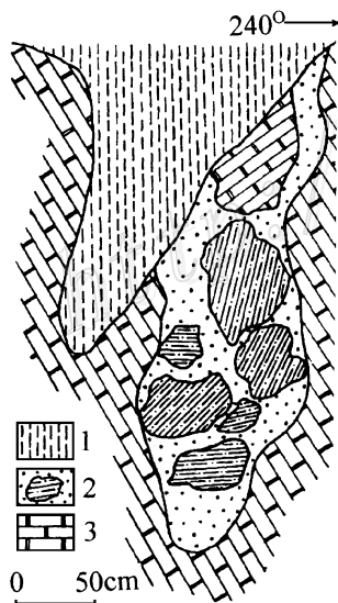
图4 上芒岗金矿麦窝坝采场岩溶漏斗剖面图
