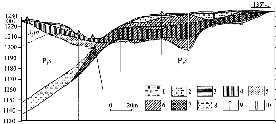
图 2 上芒岗金矿床 0 号勘探线剖面图 (据核工业云南地质调查队资料修改)
