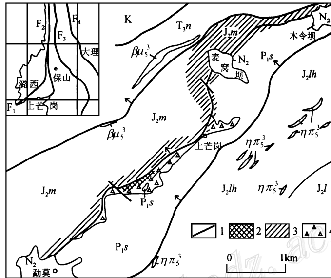
图1 上芒岗金矿床矿区地质略图
