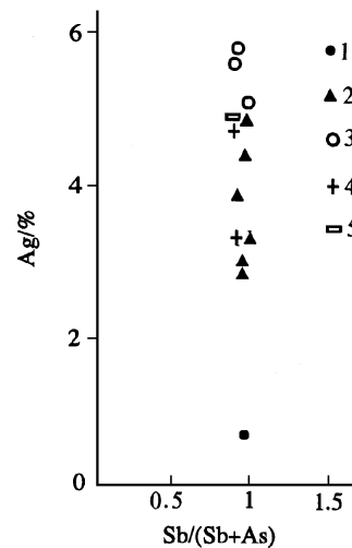
图2 夏塞矿床铜-锑-银硫盐矿物的Ag对Sb/(Sb+As)成分投绘图(原子比按(Sb+As)=4.0) 图例同图1
