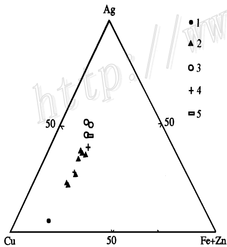
图1 夏塞矿床铜-锑-银硫盐矿物的Cu-Ag-(Fe+Zn)成分投绘图(按原子比)
