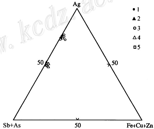
图 3 夏塞矿床 Sb-Ag 硫盐矿物的 Ag-(Sb+As)-(Fe+Cu+Zn) 成分投绘图 (按原子比)
