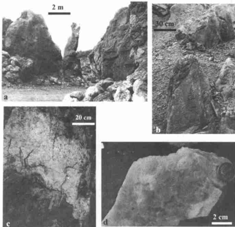
图 4 含矿碳酸盐台地的古喀斯特地貌景观和近台型 SMG 含矿硅质岩-硅质角砾岩的热水沉积特征 a—中三叠统的含金硅质岩采完后露出下伏二叠纪灰岩及其漂亮的古喀斯特地貌(广西高龙金矿); b—上二叠统大厂层含金硅质岩剥净后露出下二叠统茅口组灰岩及其古喀斯特地貌(贵州戈塘金矿); c—含矿硅质岩的热水沉积特征,包括水下侵蚀间断、角砾和纹层(详见文字描述)(贵州戈塘金矿); d— \text{SiO}_2 胶状沉积物经重结晶后形成的石英菊花状构造(广西高龙金矿)
