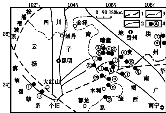
图1 滇黔桂地区卡林型金矿分布略图
