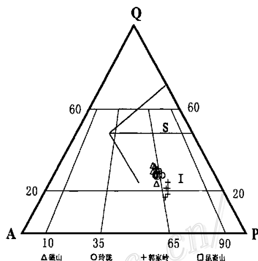
图 3 QAP 图解(据 Bowden et al., 1985) (数据见表 3)
