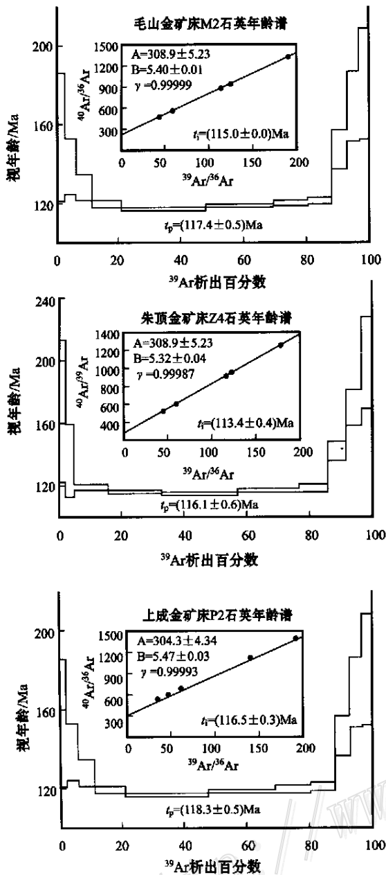
图 2 毛山、朱顶和上成金矿床石英的 40 Ar/ 39 Ar 同位素年龄谱
