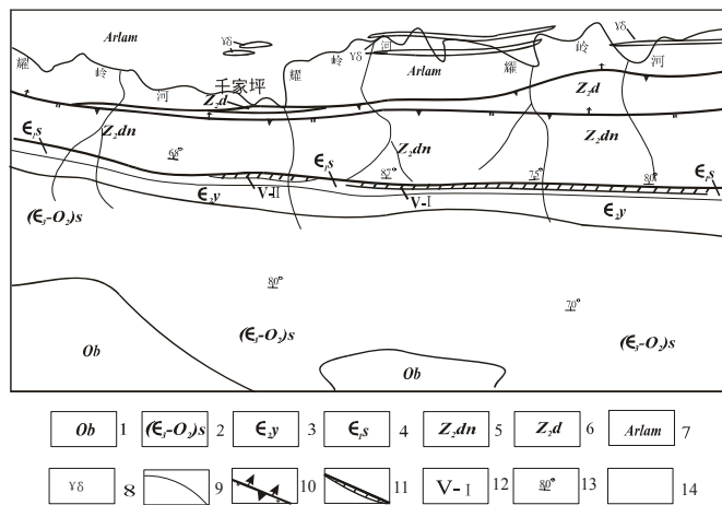
图 1 商南千家坪钒矿地质简图 (据朱红周, 2001 修编)
