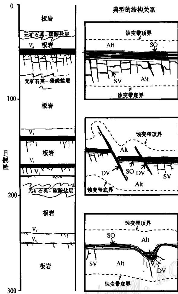
图 2 V_1 - V_6 矿体在赋矿地层中的产出位置以及层状矿石 (SO) 细脉状矿化 (SV)、切层脉体 (DV) 和围岩蚀变 (Alt) 之间结构关系示意图
