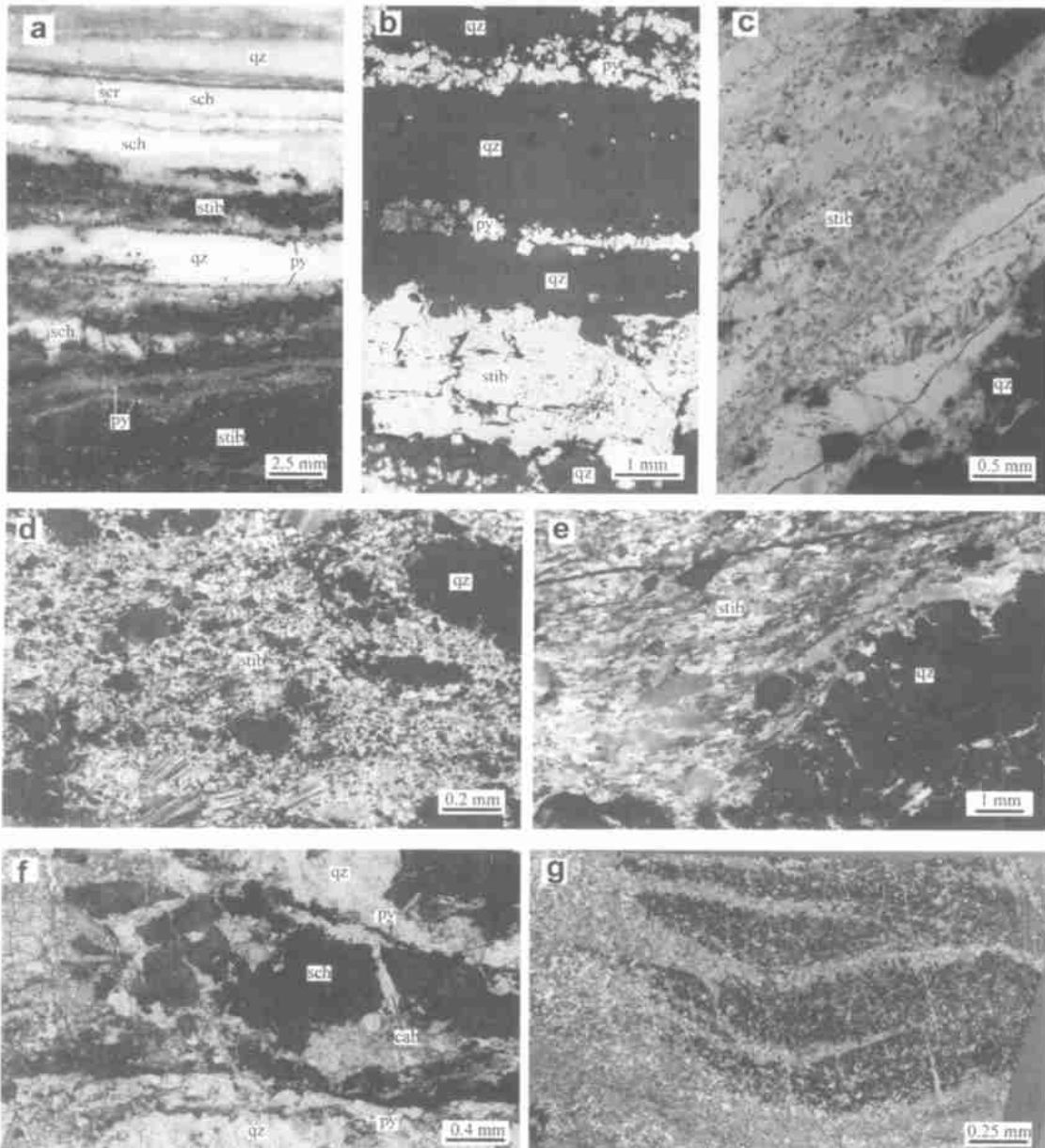
图4 典型矿石组构的显微照片
