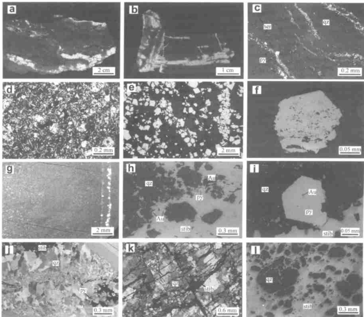
图 5 沃溪矿床的典型矿石组构
