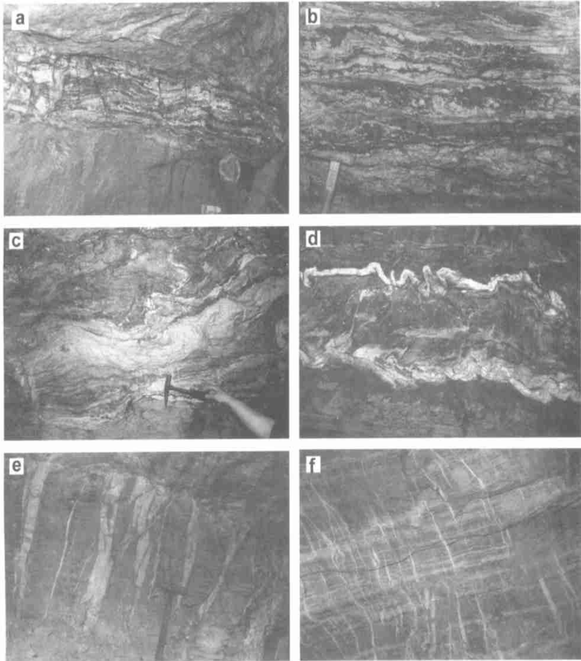
图3 沃溪矿床中两种主要矿化类型的宏观特征
