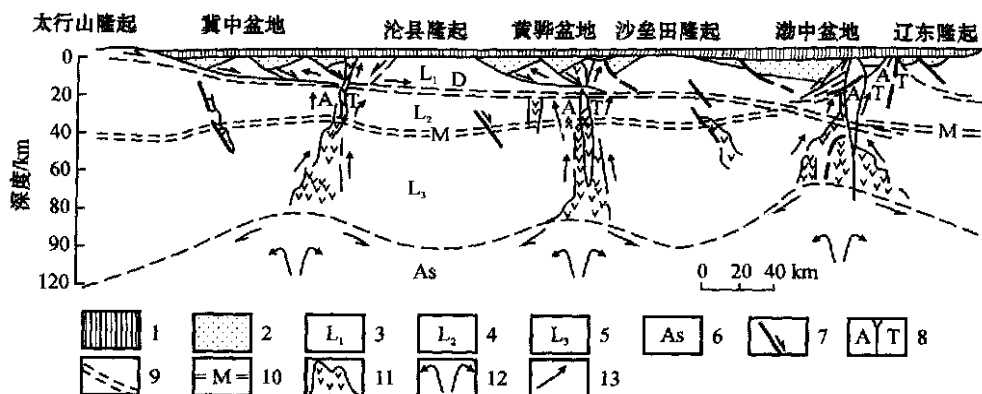
图 3 渤海湾新生代裂陷盆地的幔源岩浆 CO 2 气藏的生成模式图(据漆家福等, 1995; 陈永见, 1999)
