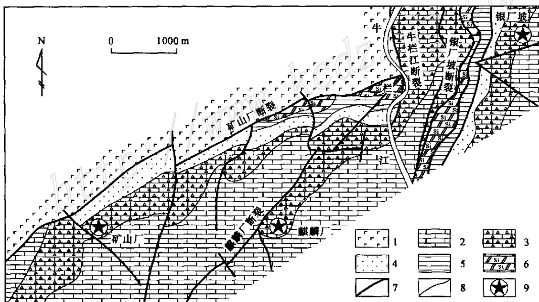
图1 云南会泽铅锌矿床地质简图(据黄智龙,2004)
