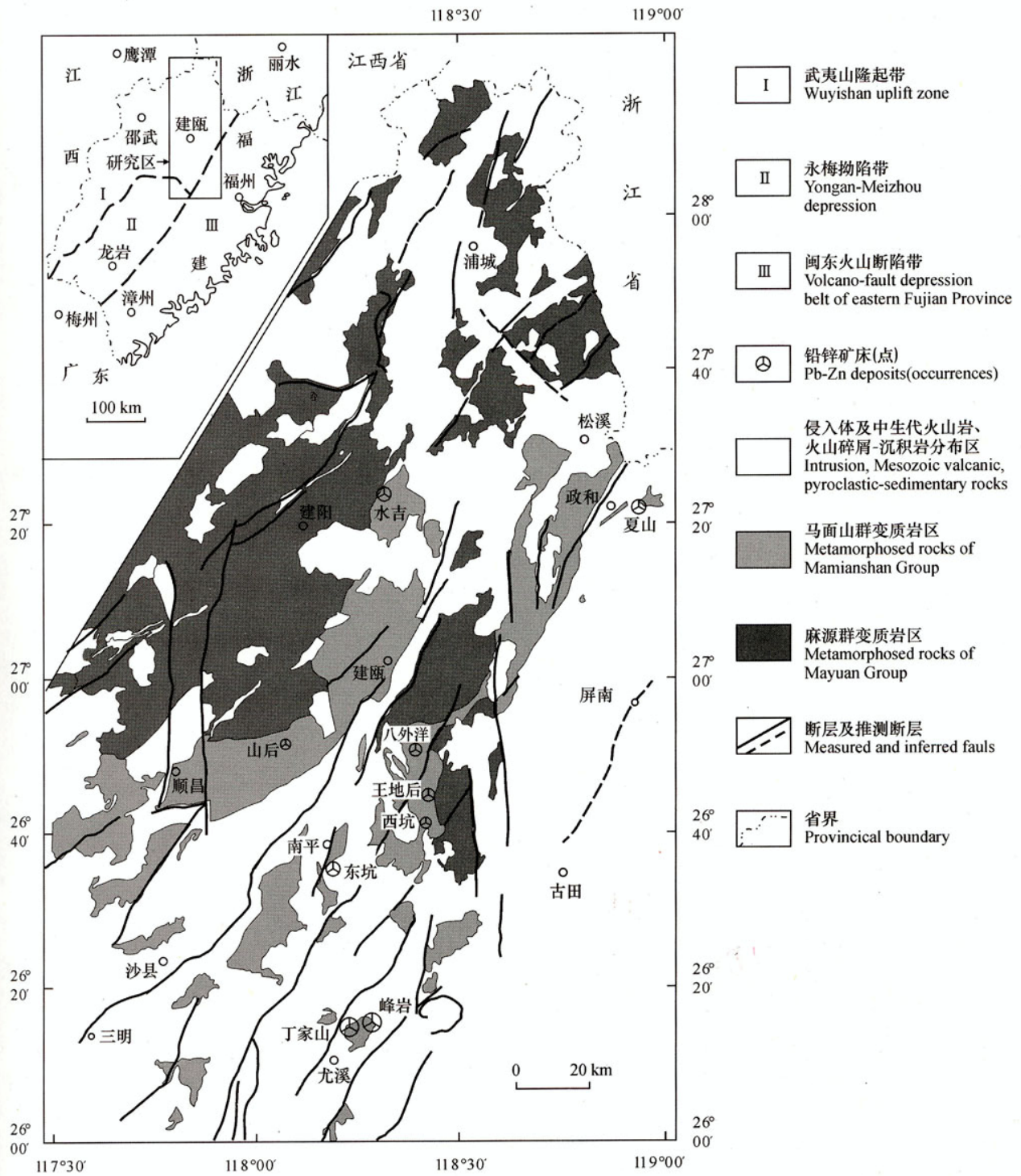
图 1 闽中地区地质构造略图(据 Zhang et al., 2004 修改)
