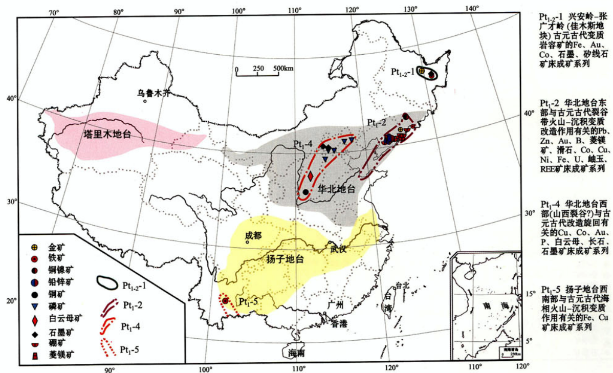
图 2 古元古代矿床成矿系列分布示意图
