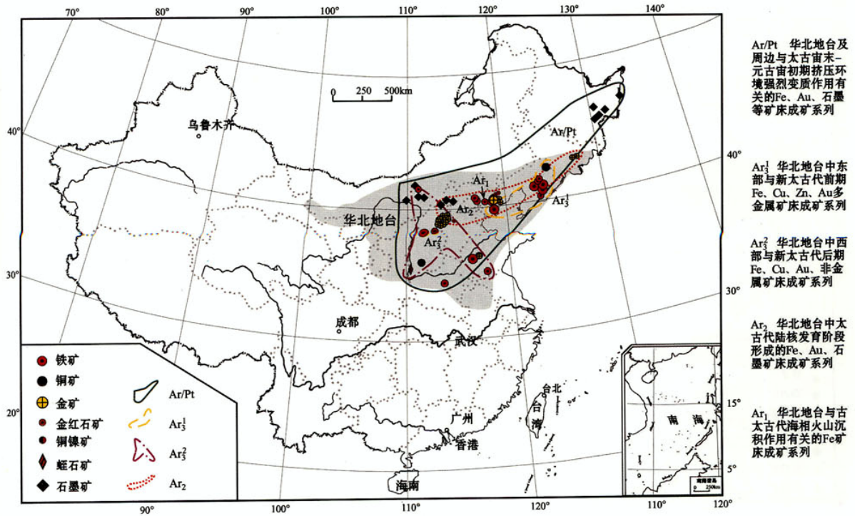
图 1 太古宙陆核阶段矿床成矿系列分布示意图
