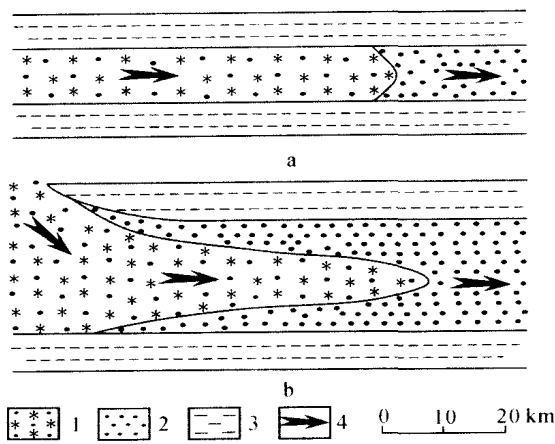
图4 典型层间氧化带(a)与潜水层间氧化带(b)模式对比示意图
