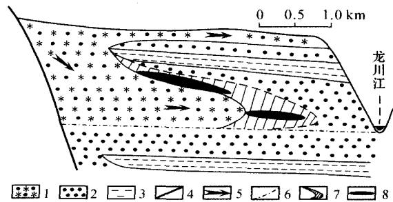
图 6 断陷带潜水层间氧化带砂岩型铀矿矿体定位模式示意图
