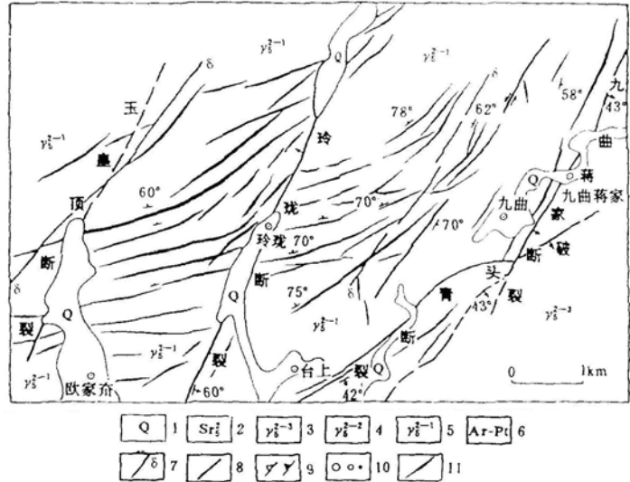
图1 玲珑金矿田地质简图
