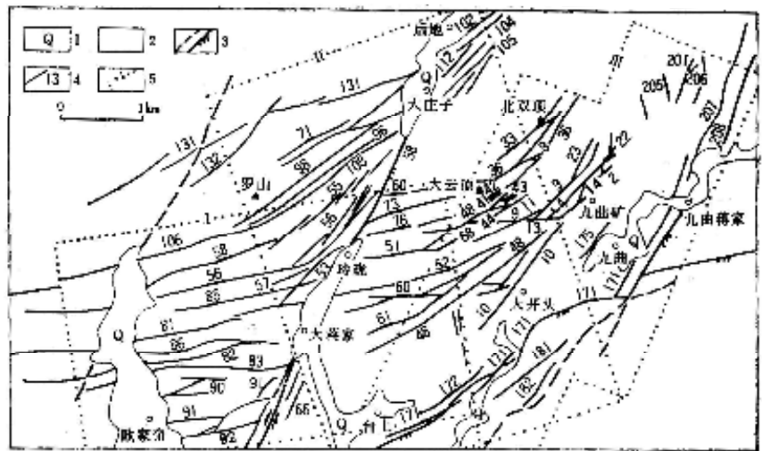
图 2 玲珑金矿田构造矿化富集带分布略图
