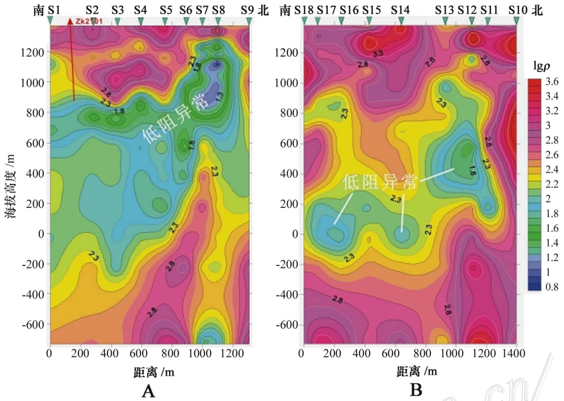
图3 图拉尔根21线 (A) 和41线 (B) 大地电磁测深 (MT) 测量结果
