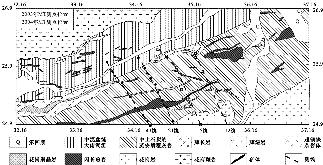
图 1 新疆哈密市图拉尔根铜镍矿地物综合图(底图据孙赫等, 2006)
