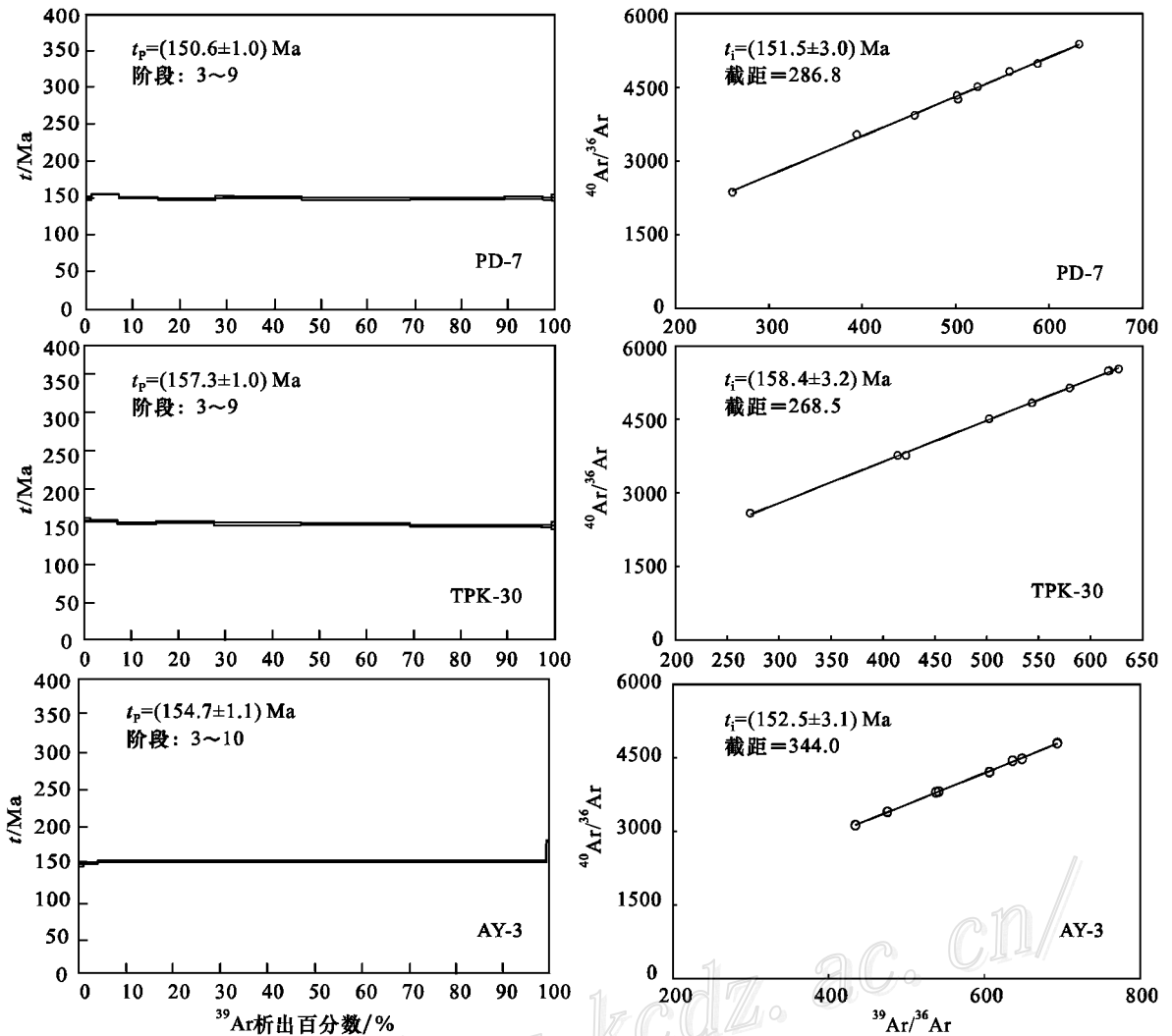
图2 芙蓉锡矿床白腊水矿区金云母的 Ar-Ar 坪年龄(左)及等时线年龄(右)
