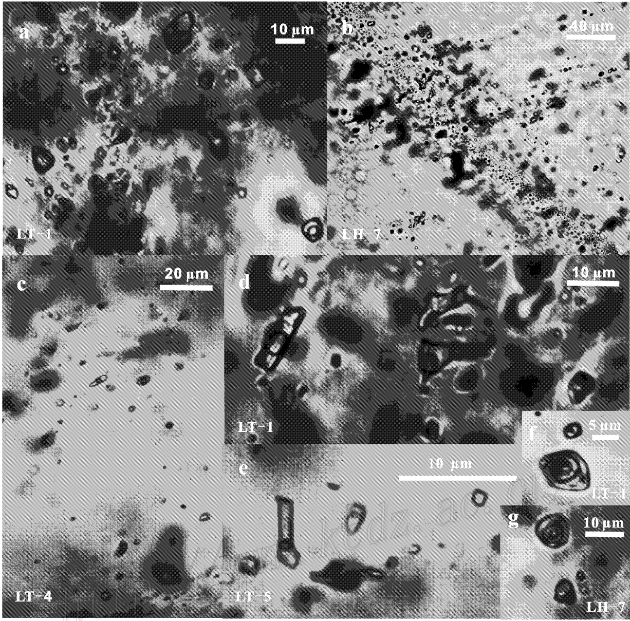
图 5 六合坳和烂头山矿石包裹体照片
