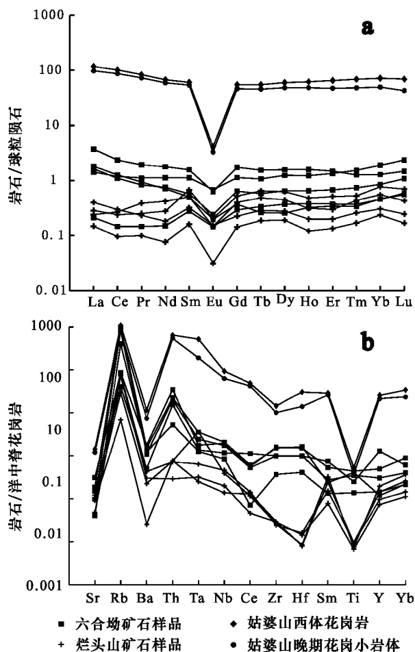
图3 六合坳矿石、烂头山矿石、姑婆山西体花岗岩及晚期花岗岩小岩体的REE配分图(a)和不相容元素的洋中脊花岗岩标准化蛛网图(b) 球粒陨石标准化值据 Taylor 等(1985); ORG 值据 Pearce (1982, 1983)
