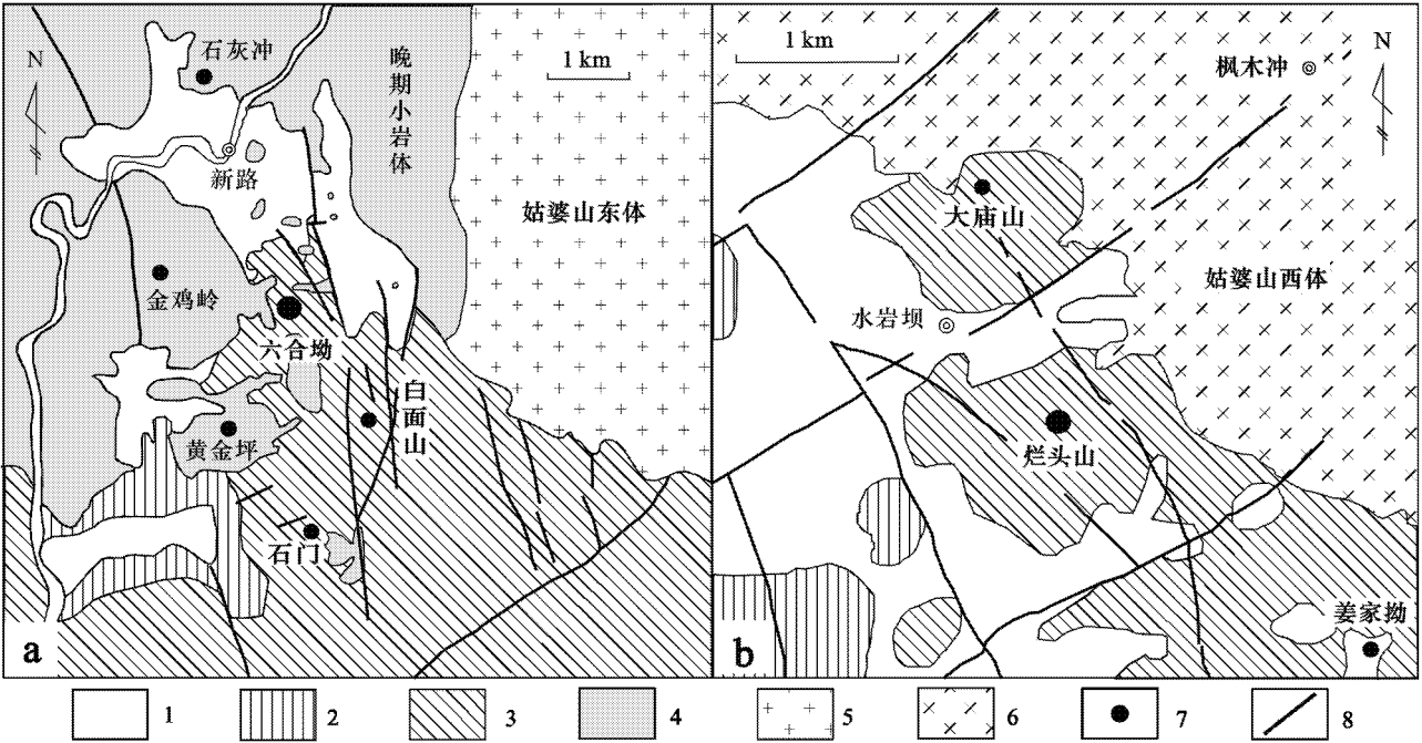
图 2 广西新路(a)和水岩坝(b)矿地质简图(据董子成,1991;谢国源等,1994 资料改编)
