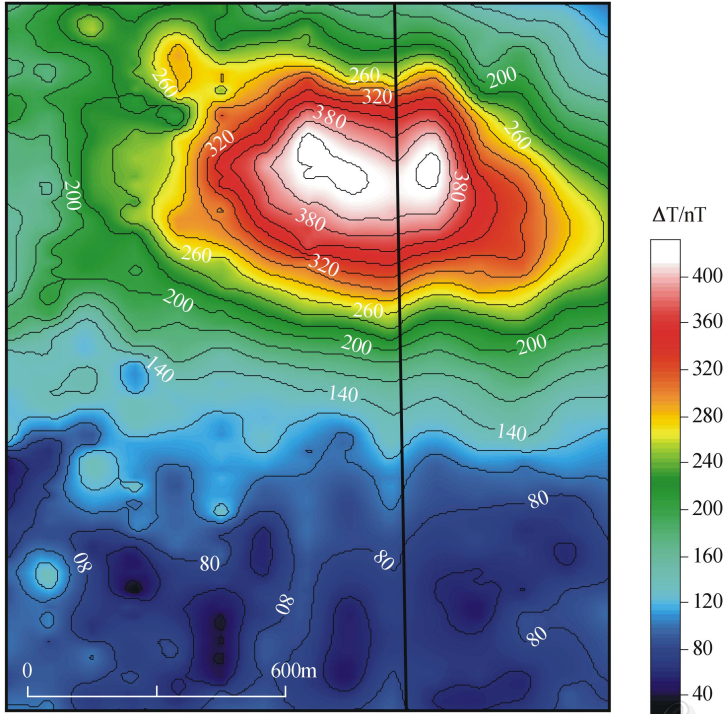
图 7 羊蹄子山-磨石山矿区马牙子山 M1 化极磁异常图
