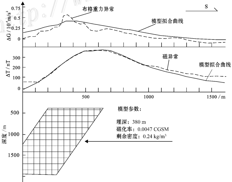
图 8 羊蹄子山-磨石山矿区马牙子山 M1 磁异常 178 线反演解释剖面图
