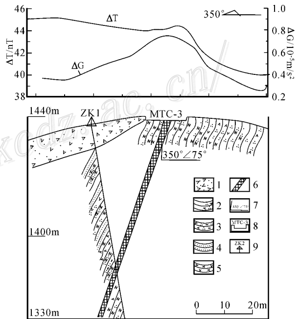
图4 磨石山矿床第6勘探线物探-地质综合剖面 (地质剖面据①修改)
