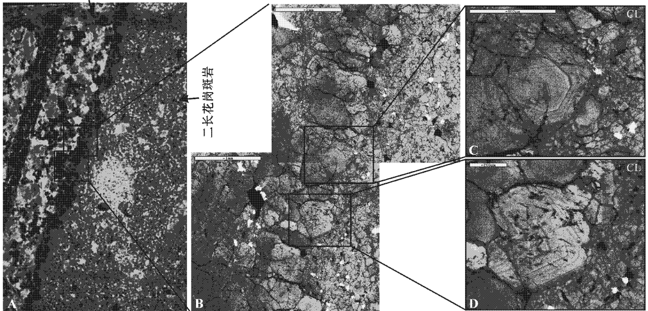
花岗闪长岩
