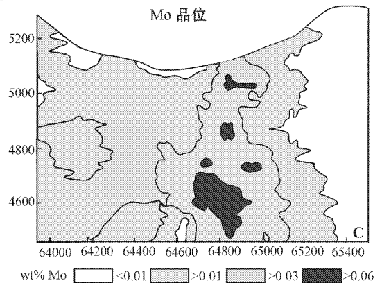
图 10 驱龙铜矿典型剖面蚀变分带及该剖面 Cu、Mo 分布等值线图, 显示蚀变与矿化的关系 (据 Yang et al., 2009 修改)
