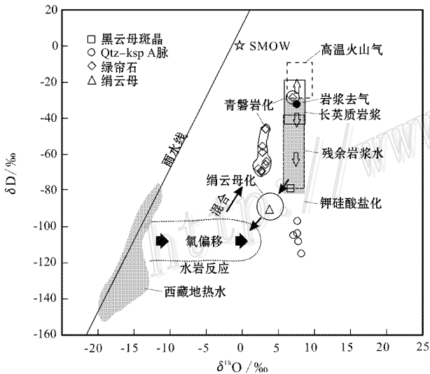
图 14 驱龙铜矿与各期蚀变有关流体的 \delta D-\delta^{18}O 模式图(杨志明, 2009)。雨水通常会因在流动过程中发生水岩反应造成氧同位素偏移(Hedenquist et al., 1994)
