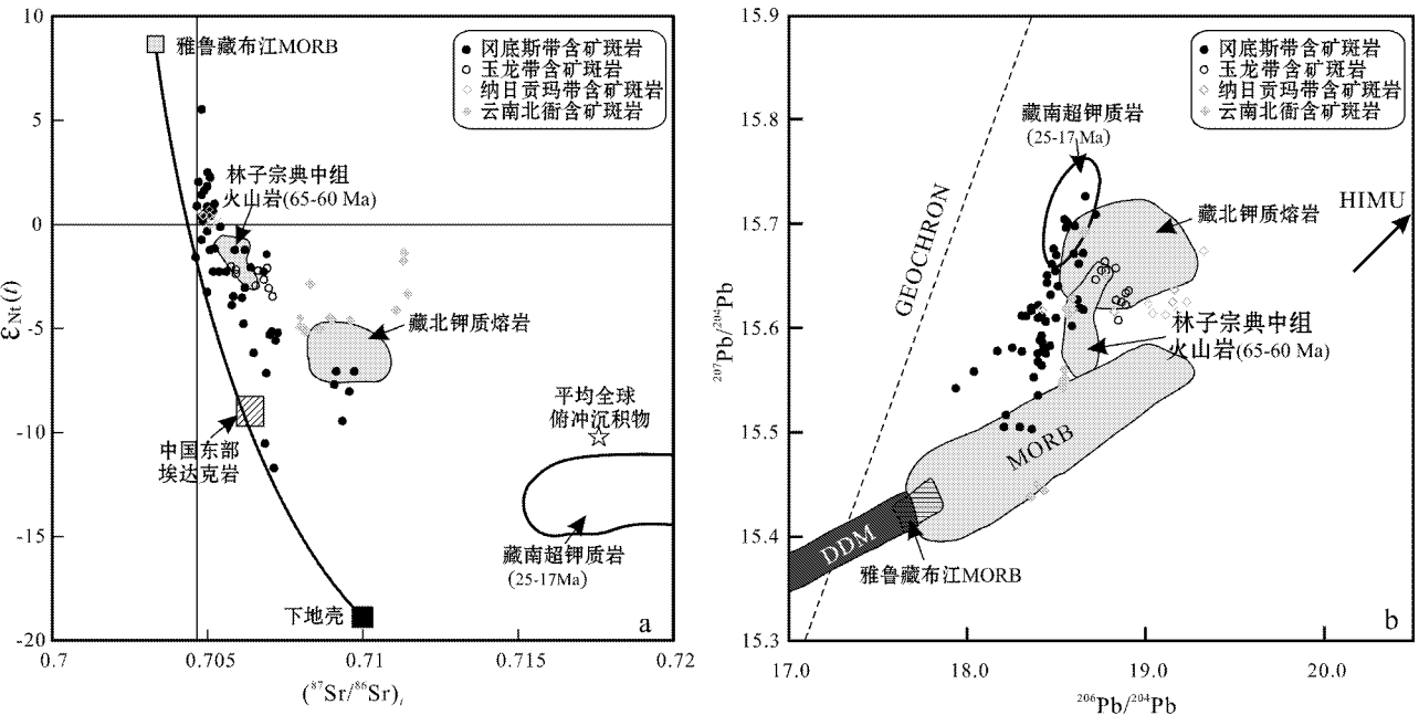
图 8 青藏高原典型斑岩铜矿带含矿斑岩 87 Sr/ 86 Sr- 143 Nd/ 144 Nd (a)及 207 Pb/ 204 Pb- 206 Pb/ 204 Pb (b)图解
