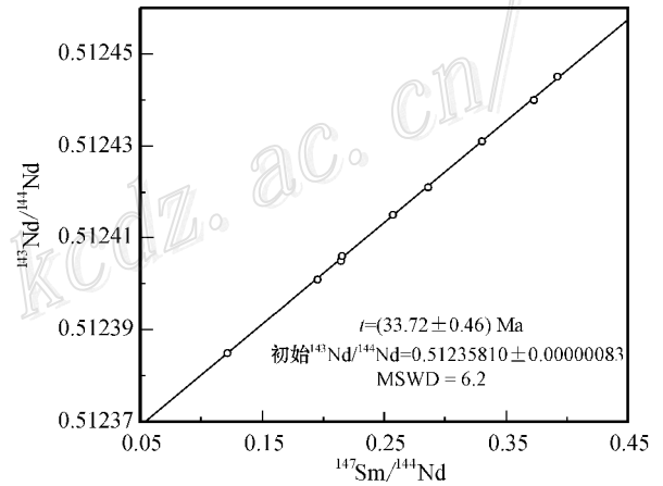
图 8 莫海拉亨铅锌矿床共生矿物组合萤石与方解石 Sm-Nd 等时线图
