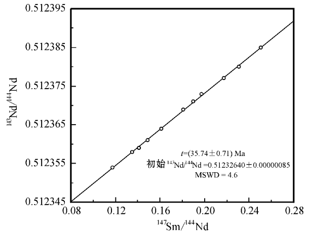
图4 东莫扎抓铅锌矿床共生矿物组合闪锌矿与黄铁矿 Sm-Nd 等时线图
