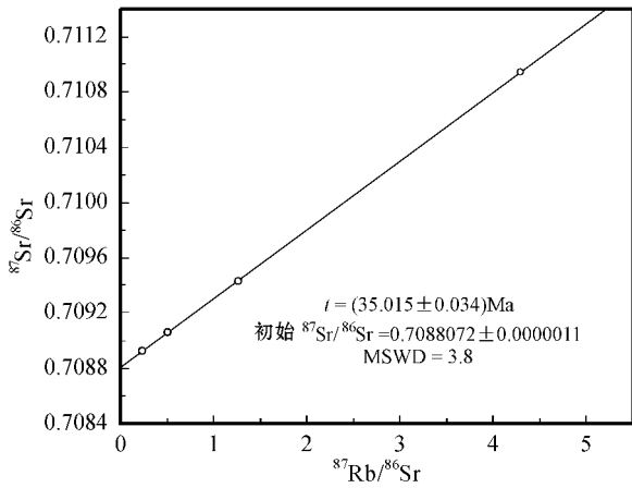
图2 东莫扎抓铅锌矿床闪锌矿 Rb-Sr 等时线图
