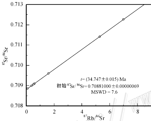
图3 东莫扎抓铅锌矿床共生矿物组合黄铁矿与方铅矿 Rb-Sr 等时线图
