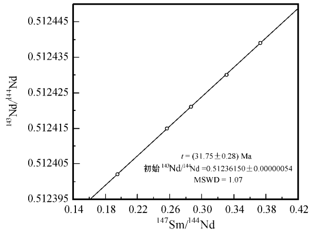
图 7 莫海拉亨铅锌矿床萤石 Sm-Nd 等时线图
