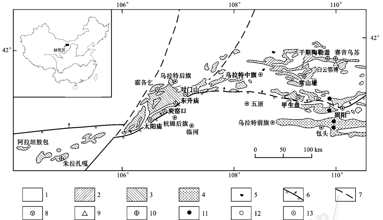
图 1 内蒙古中西部重要金属矿床分布简图(根据胡鸿飞等 2008 和 黄占起等 2002 资料改编)
