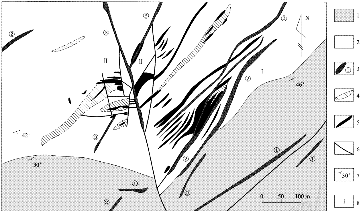
图2 朱拉扎嘎金矿床地质简图(根据 Jiang et al., 2005 资料改编)
