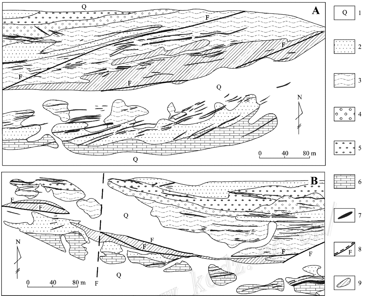
图4 常山壕金矿床地质简图(据宁夏核工业地质勘查院 2005 资料 ① 改编)
