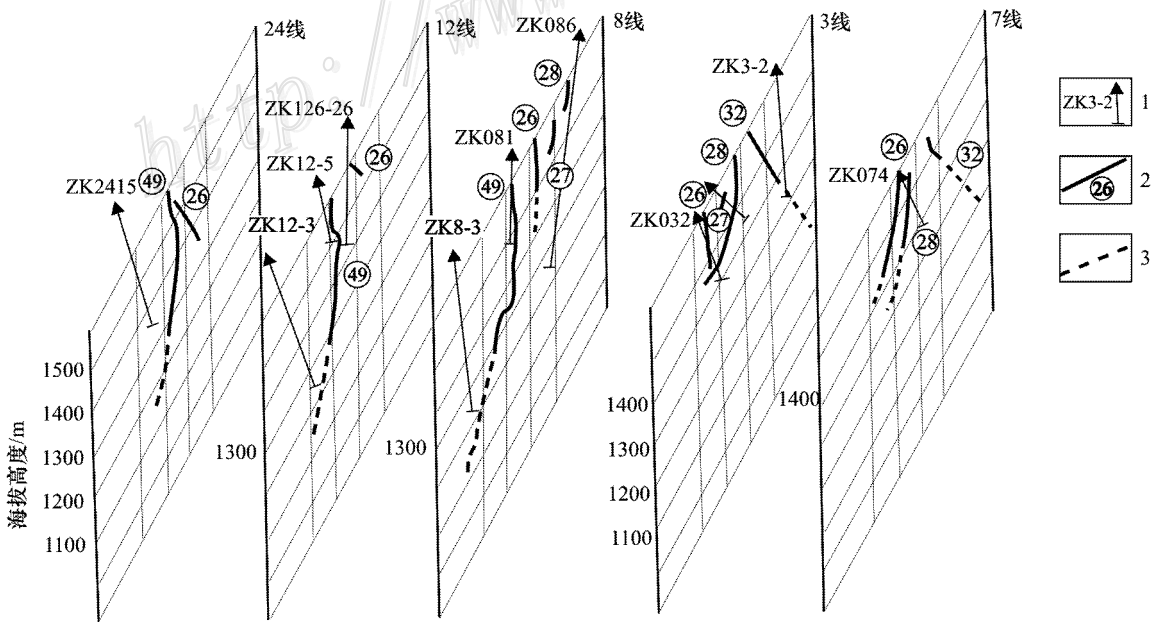
图7 赛音乌苏金矿床代表性地质勘探剖面简图(据张学权等2007资料改编)
