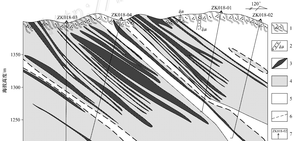
图3 朱拉扎嘎金矿床 P018 地质勘探线剖面图(根据 Jiang et al., 2005 资料改编)
