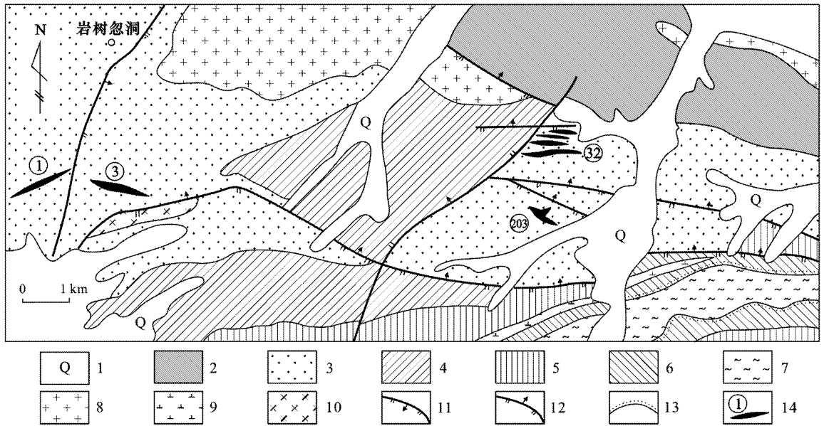
图6 赛音乌苏金矿床地质简图(据张学权等2007资料改编)
