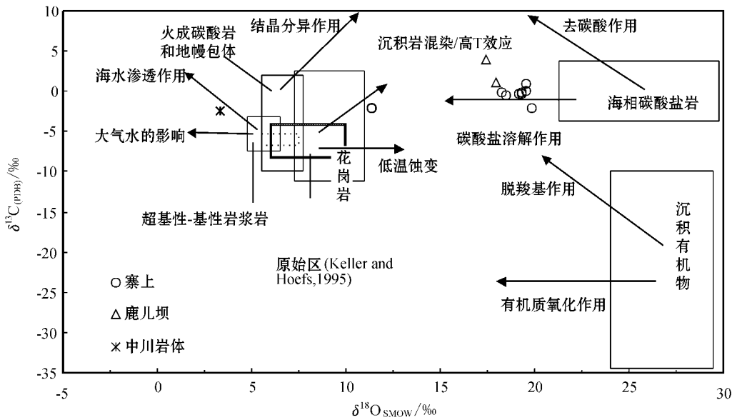
图 9 寨上金矿床中方解石和菱铁矿的 \delta^{18}\text{O} - \delta^{13}\text{C} 图解
