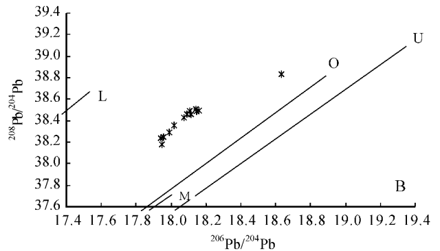
图7 寨上金矿床铅构造模式图(底图据 Doe et al., 1979; Zartman et al., 1981)
