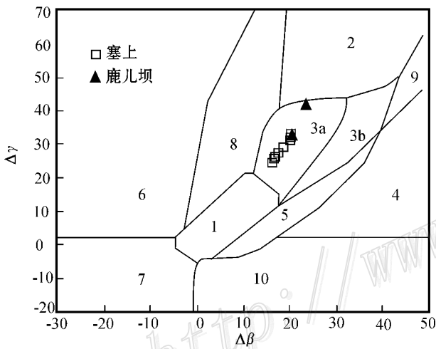
图8 寨上金矿床矿石、围岩铅同位素的 \Delta\beta - \Delta\gamma 成因分类图解(底图据朱炳泉, 1998)
