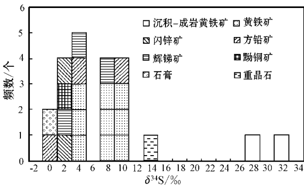
图 6 寨上金矿床硫同位素组成分布图
