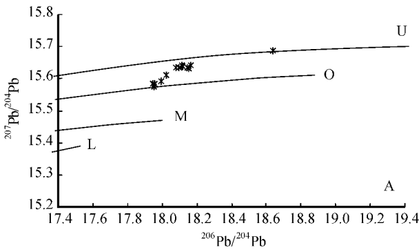
图7 寨上金矿床铅构造模式图(底图据 Doe et al., 1979; Zartman et al., 1981)
