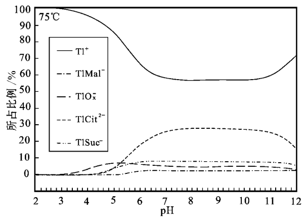
图4 在 75°C 氧化环境中铊的诸物种在不同 pH 值条件下的分配
