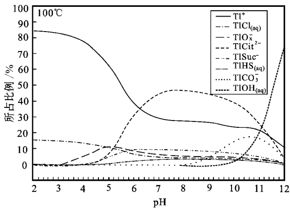
图2 在 100°C 氧化环境中铊的诸物种在不同 pH 值条件下的分配
