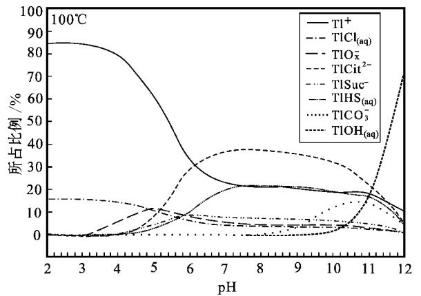
图 1 在 100℃ 还原环境中铊的诸物种在不同 pH 值条件下的分配
