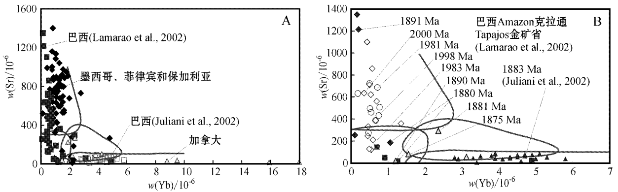
图7 国外与金和金铜矿床有关的花岗岩的 Sr-Yb 图(A)和巴西 Tapajos 金矿省花岗岩和火山岩的 Sr-Yb 图(B)
