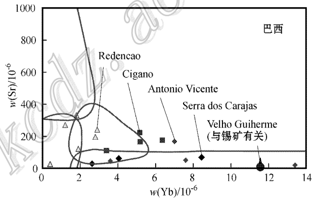
图 15 巴西古元古代花岗岩的 Sr-Yb 图
