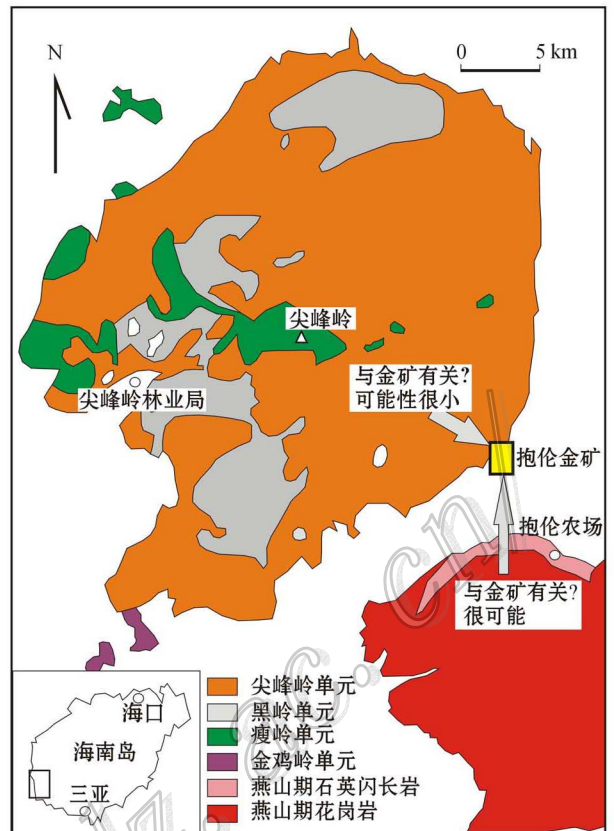
图20 海南尖峰岭花岗岩和抱伦金矿地质图 (据张小文等,2009简化)
