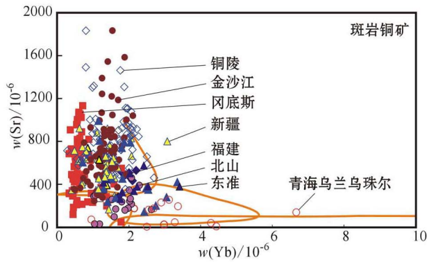
图3 中国若干斑岩铜矿的斑岩的 Sr-Yb 图
