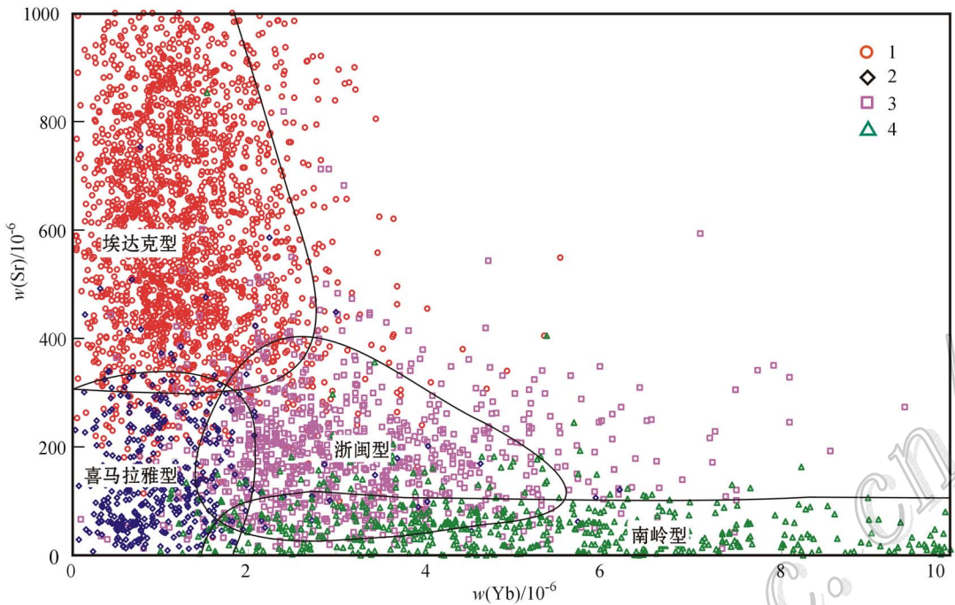
图 1 花岗岩按照 Sr-Yb 含量的分类(张旗等, 2010)
