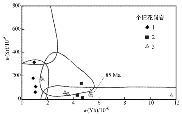
图 13 个旧花岗岩 Sr-Yb 图
