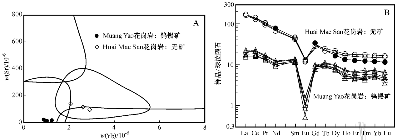
图 14 泰国 Khuntan 岩基的 Sr-Yb 图 (A) 和 REE 分布图 (B) (Yokart et al., 2003) 球粒陨石标准化值引自 Sun 等, 1989
