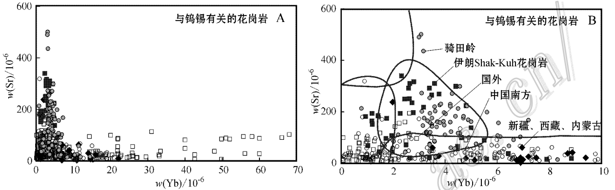
图 12 与钨锡成矿有关的花岗岩的 Sr-Yb 图
