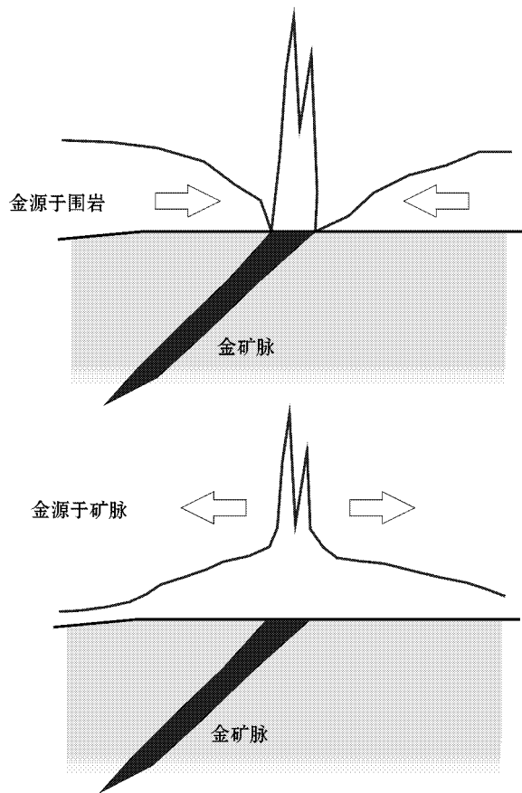
图 19 两种可能的 Au 异常剖面图
