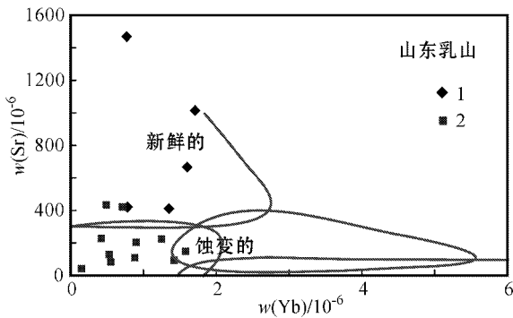
图 6 山东乳山金矿新鲜的和蚀变的花岗岩的 Sr-Yb 图 (资料据凌洪飞等,2002)
