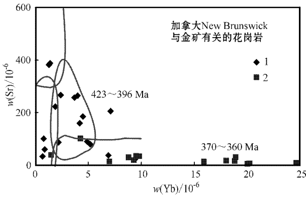
图 8 加拿大 New Brunswick 与金矿有关的花岗岩的 Sr-Yb 图(资料据 Yang et al., 2008)
