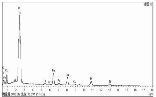
图 8 主要金属矿物扫描电镜图像与电镜能谱分析谱线图(2)
