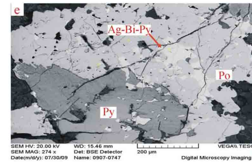
图 8 主要金属矿物扫描电镜图像与电镜能谱分析谱线图(1)
