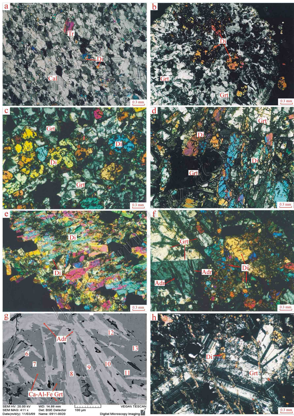
图 5 典型矽卡岩、石榴子石与透辉石显微照片
