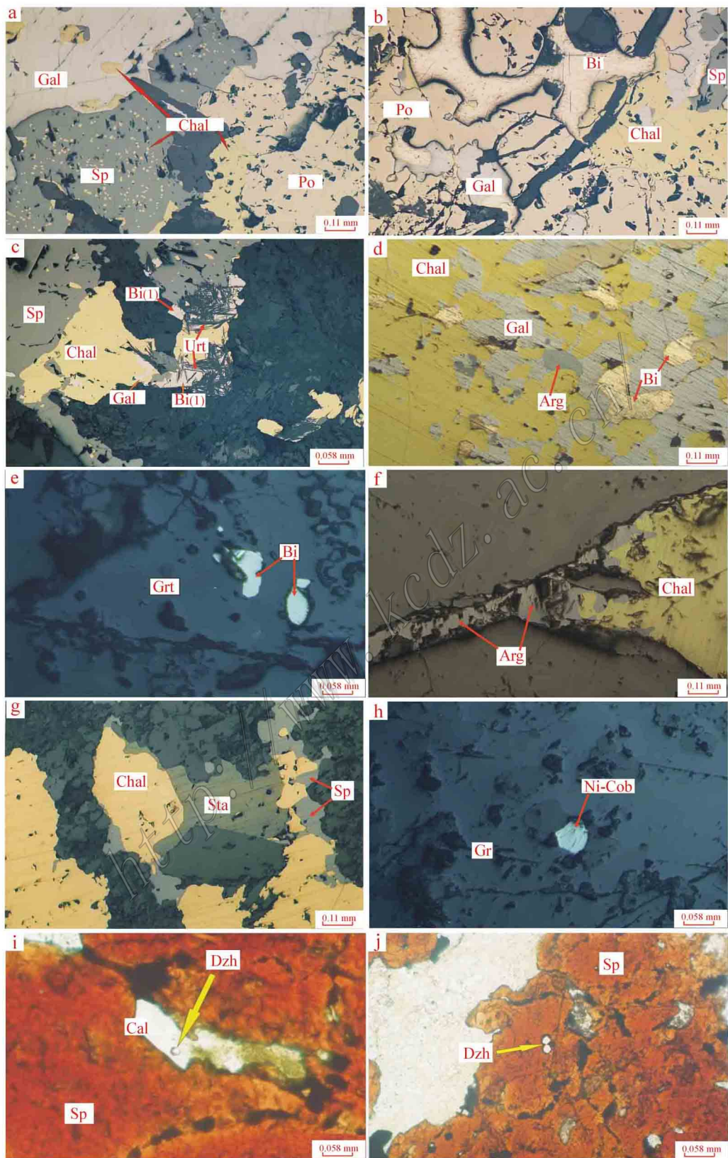
图7 拉屋矿区金属矿物显微照片
