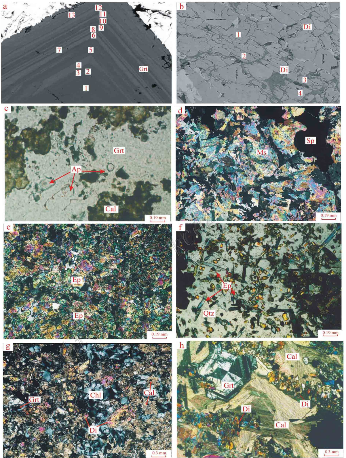
图 6 典型蚀变岩石显微照片
