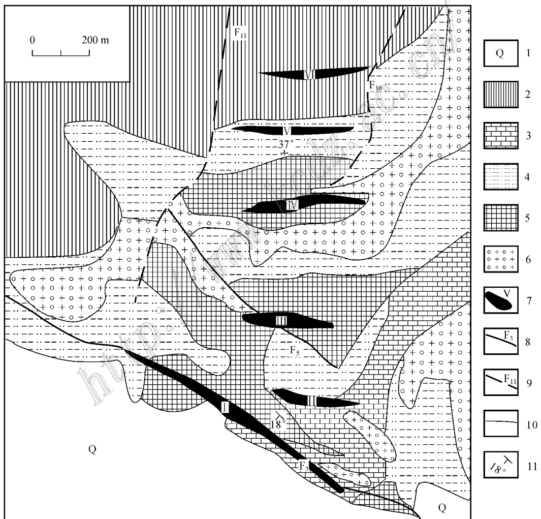
图 2 拉屋矿区地质图(据刘延勇,2008,修改)
