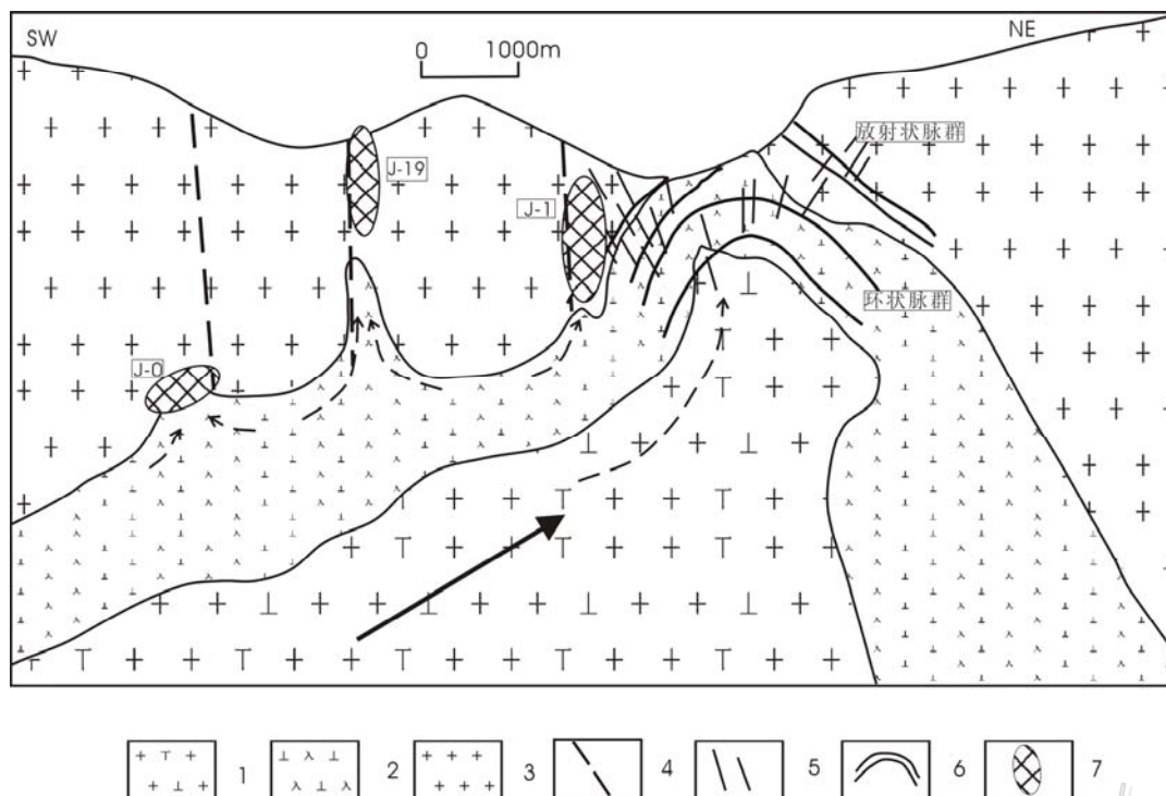
图6 金厂矿区构造控矿剖面模式图
