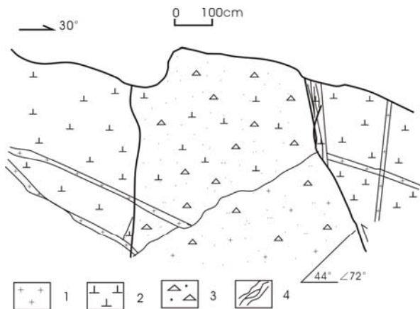
图 2 近 NW 向断裂构造素描图
