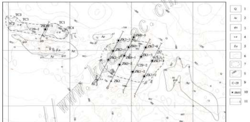
图1 大西沟铁磷矿区磁异常及地质略图
