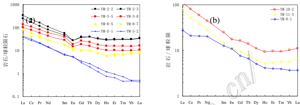
图2 油麻坡钨钼矿岩石、矿石矿物稀土元素配分模式图
