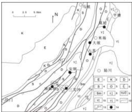
图1 博白县油麻坡钨钼矿床区域地质略图
