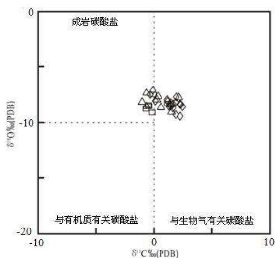
图 1 胶结物成因碳、氧同位素判别图 (底图据王大锐, 2000)
