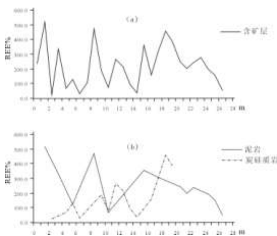
图 2 千家坪矿区矿层稀土总量( \Sigma REE)变化曲线图
