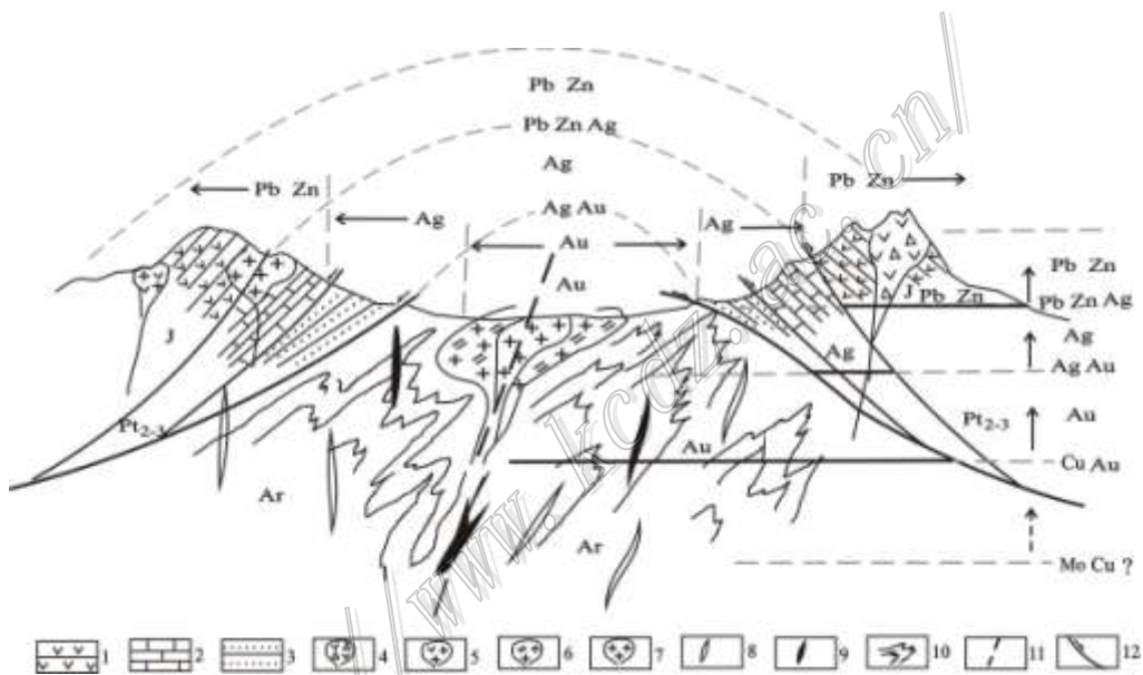
图2 张宣幔枝构造区深部成矿模式图
