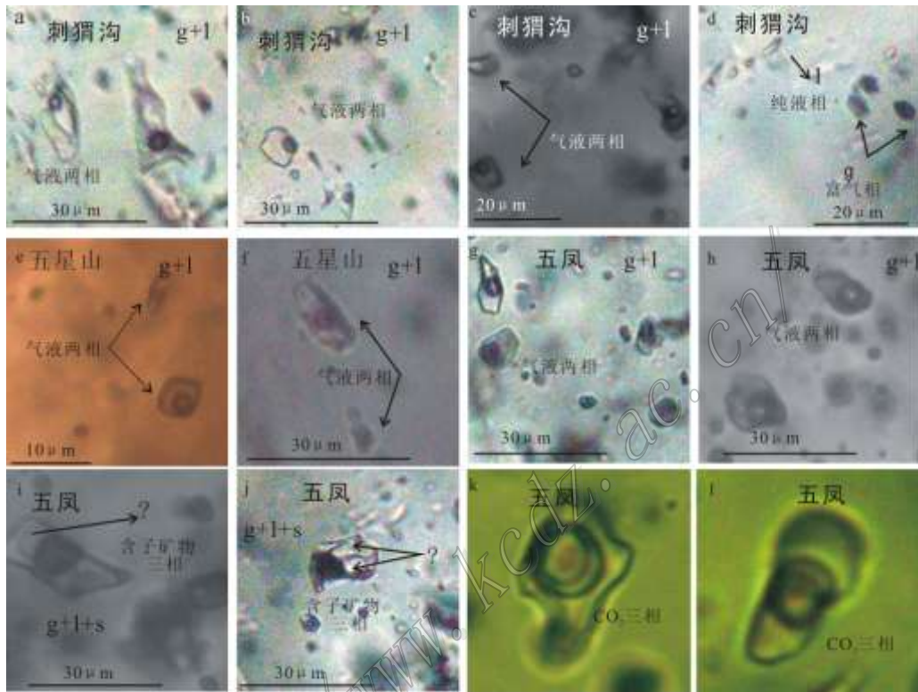
图1 延边地区典型低硫化热液金矿床典型包裹体照片
