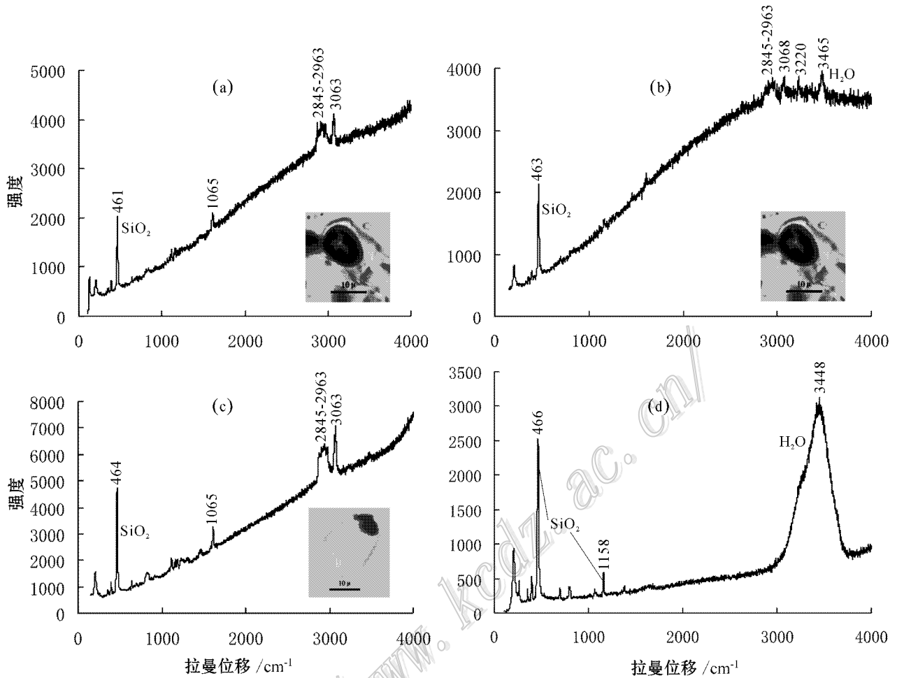
图5 沙子江铀矿床流体包裹体激光拉曼光谱
