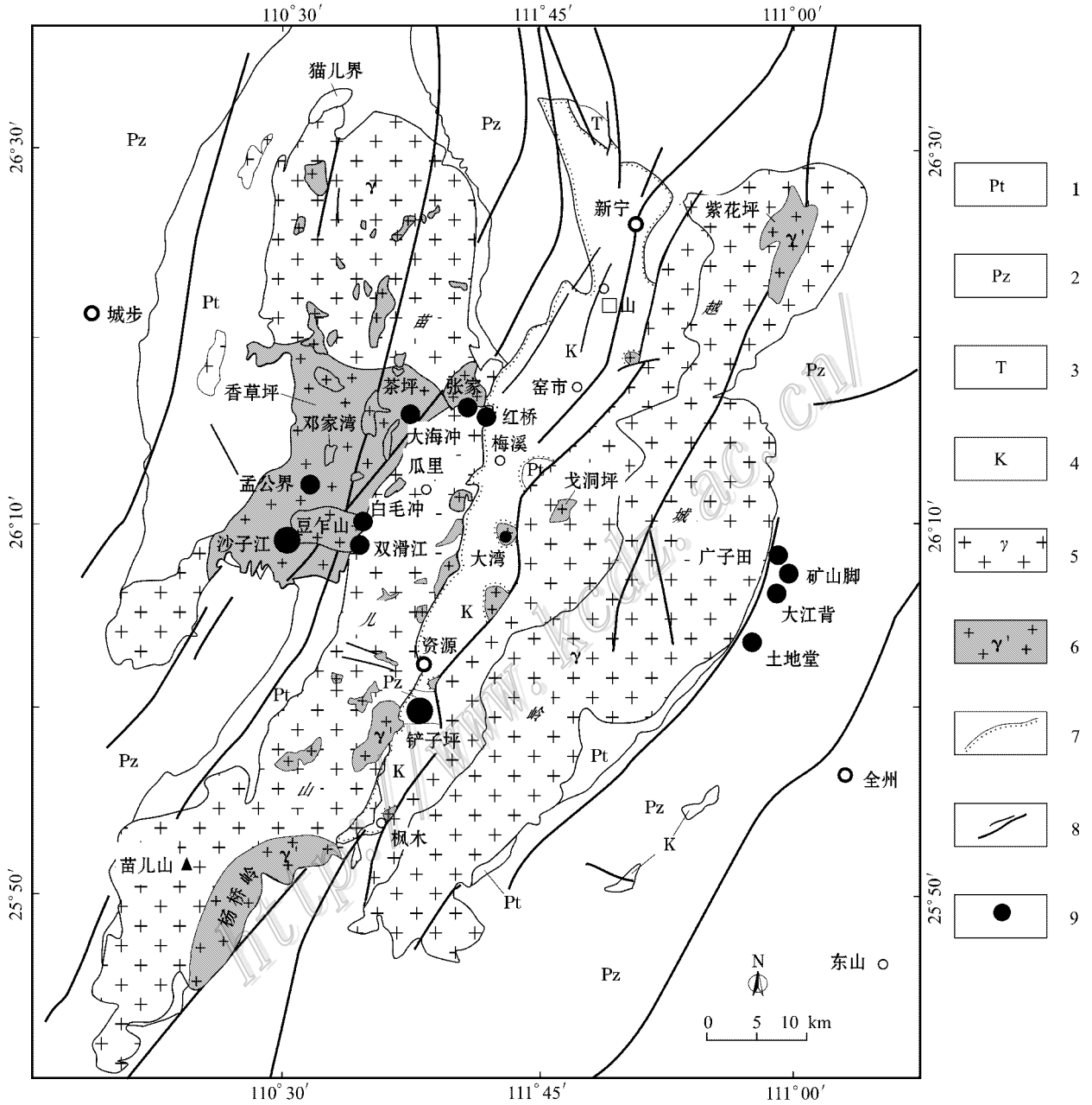
图 1 苗儿山铀成矿区地质略图(据方适宜等,2007;孙涛等,2007及广西 310 核地质大队,1991 ① 综合)
