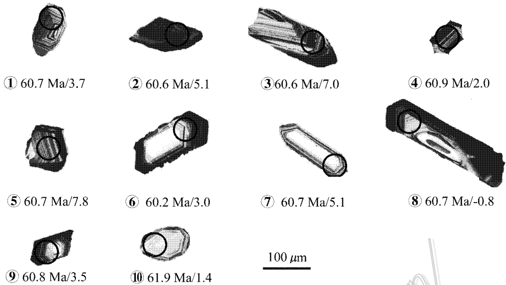
图5 邦铺矿床黑云二长花岗岩锆石阴极发光图像 测试点位分析点下的数字表示 U-Pb 年龄/ \epsilon_{\text{H}}(t) 值
