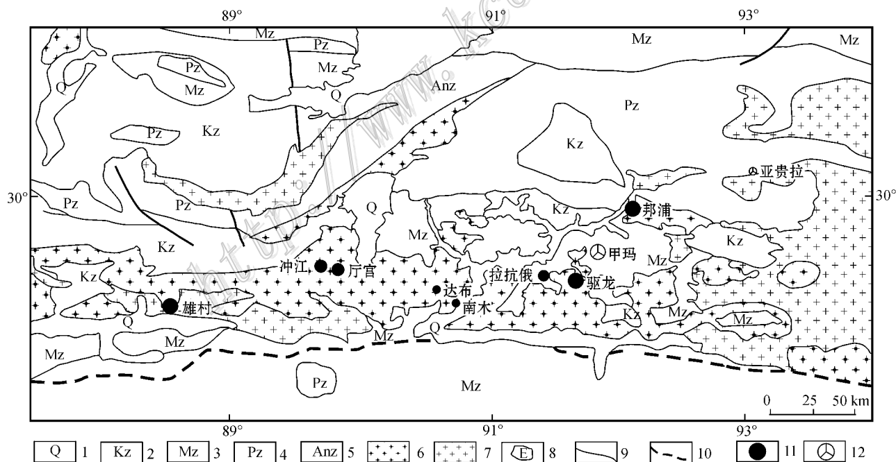
图 1 西藏冈底斯成矿带东段主要铜多金属矿床分布图(据李光明等 2005 和高一鸣 2010 修改)
