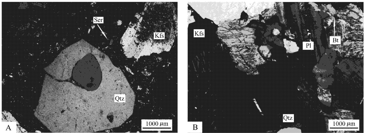
图3 石英熔蚀结构(A)及钾长石条纹结构(B)
