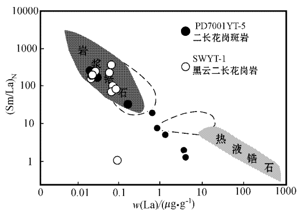
图7 锆石的 La/(Sm+La)_N 图解(底图据赵振华, 2010 修改)
