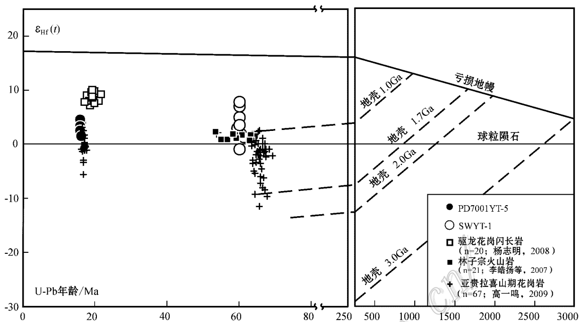
图 8 样品 PD7001YT-5(二长花岗斑岩)和 SWYT-1(黑云二长花岗岩)的锆石 Hf 同位素组成和 U-Pb 年龄作图 (底图据杨志明, 2008 和高一鸣, 2010 修改)
