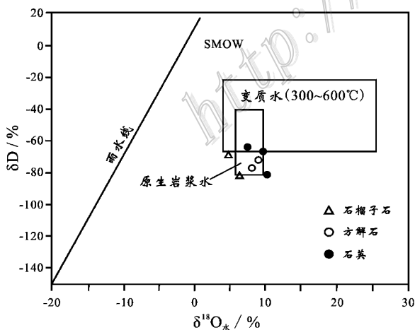
图 9 南秧田钨矿床的 \delta\text{D} - \delta^{18}\text{O}_{\text{H}_2\text{O}} 图解 (原生岩浆水范围据 Sheppard, 1986)
