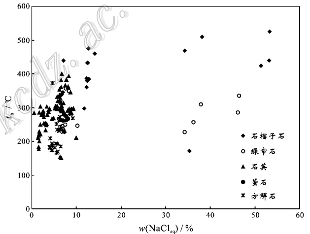
图 8 南秧田钨矿床流体包裹体的均一温度-盐度关系图
