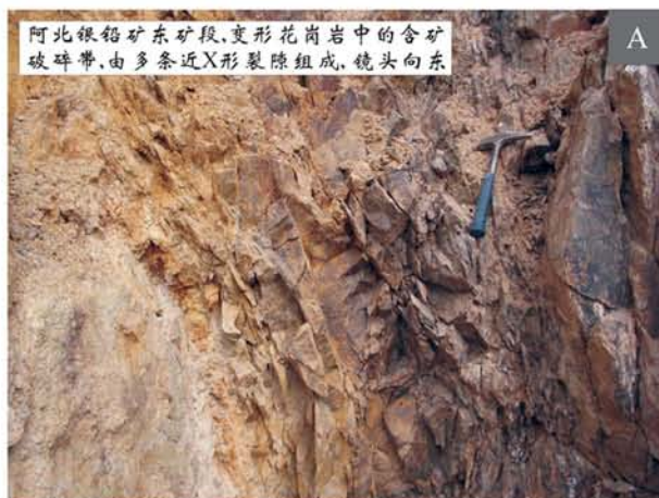
图7 阿北银铅矿东矿段控矿构造裂隙照片(H09地质点)
